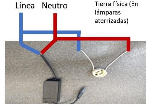
6. Realizar la conexión de la base o Driver de la lámpara a la energía eléctrica (Verificar características técnicas de la lámpara utilizada)
